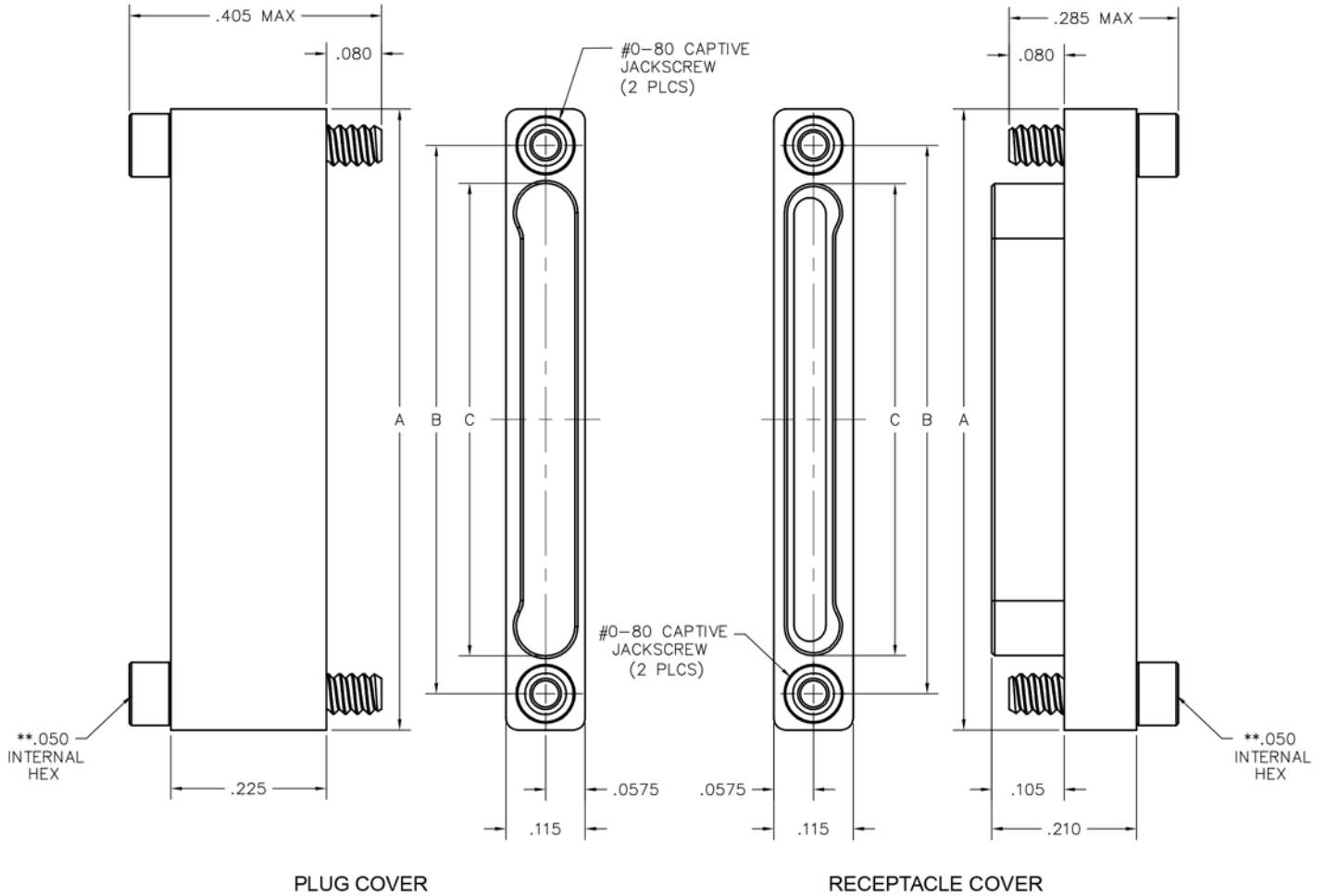
ND-1P2-025-JC (METAL)
