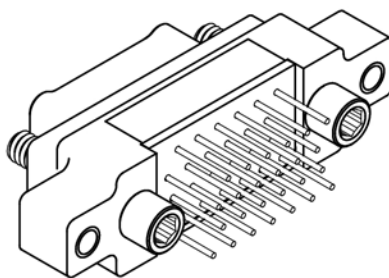
NK-2M2-025-135-JC00 PLUG
