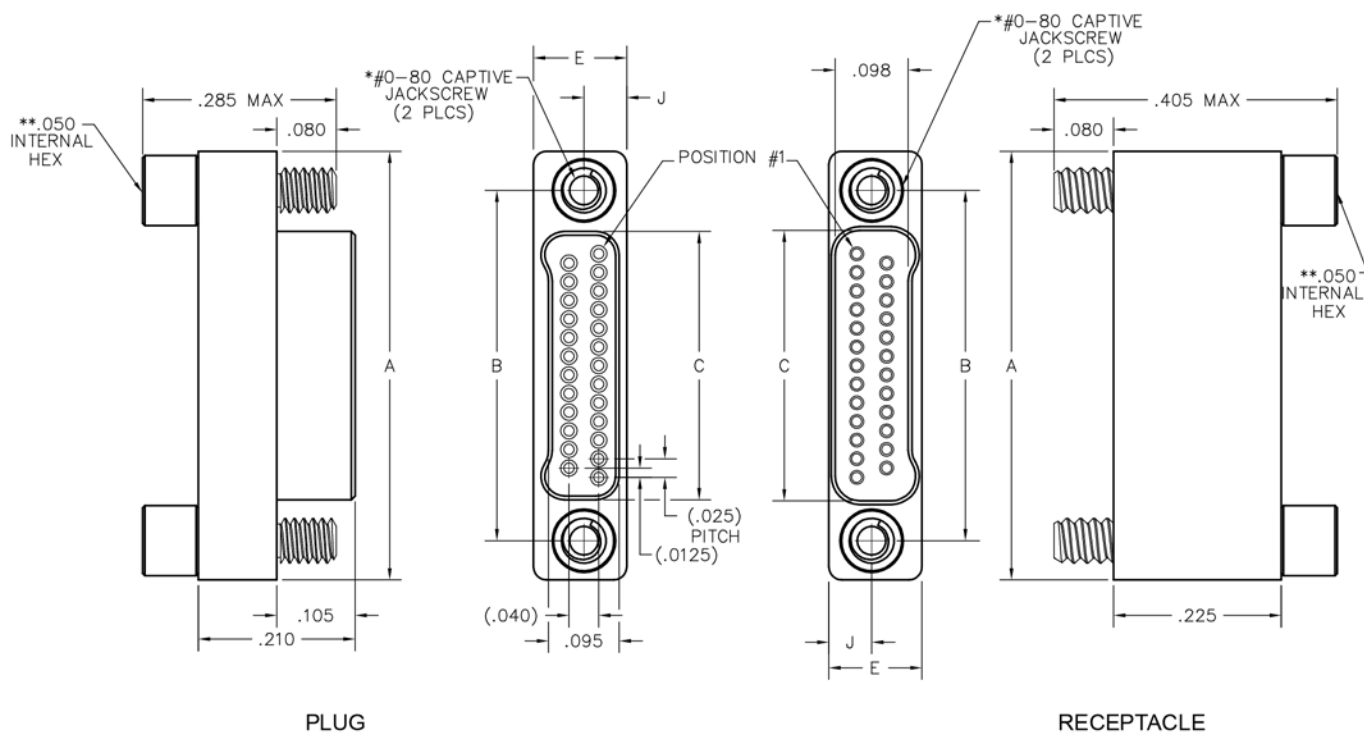
NMSH-212-025-125-JC00 (METAL)
