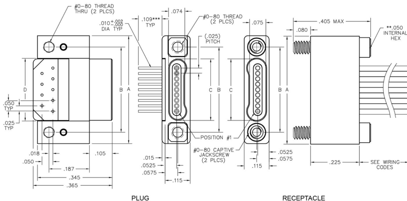
NM-122-009-261-JCAC (METAL)
