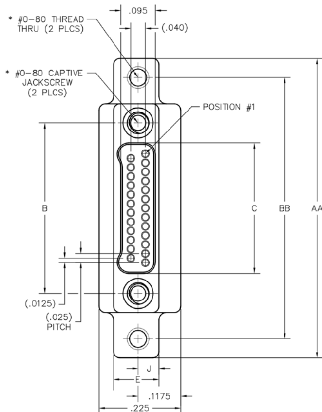
NK-2M2-025-135-JC00 PLUG
