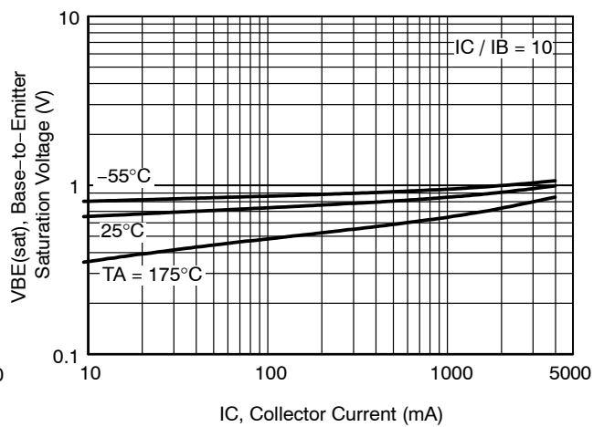
Figure 7. VBE(sat) – IC
