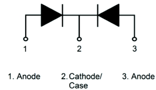
Schottky Diode
