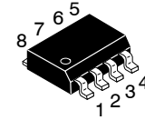
SOIC8 (SO-8) CASE 751EB
