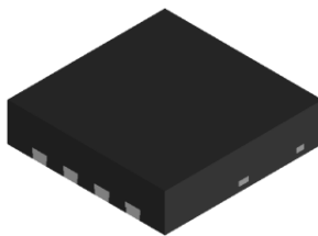
MLP 3.3x3.3
