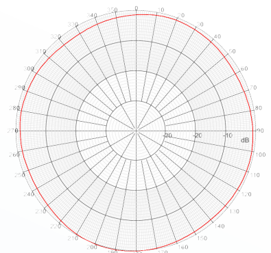
H-plane 3.55 GHz
