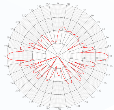
E-plane 3.55 GHz
