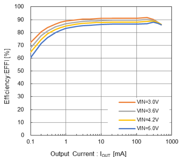
XCL242 V_{OUT(T)}=3.3V
