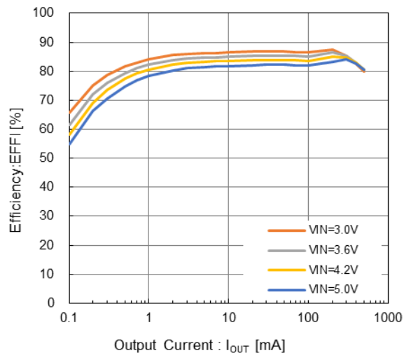
XCL242 V_{OUT(T)}=1.8V
