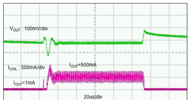
XCL242
