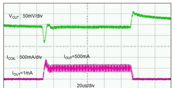
XCL242
