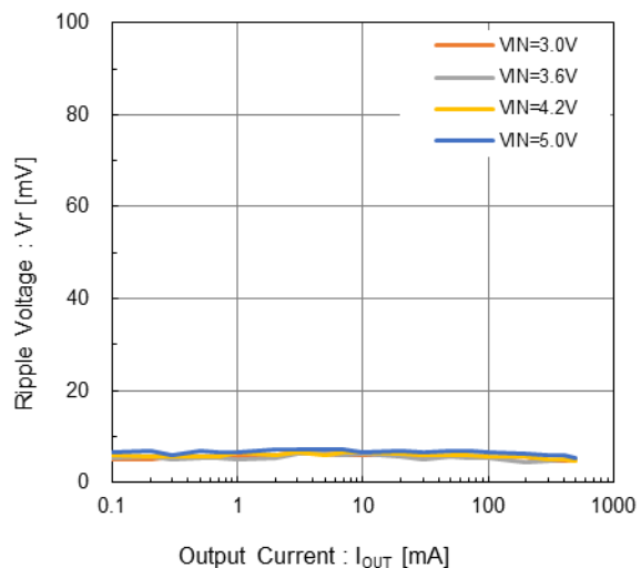
XCL241 V_{OUT(T)}=3.3V
