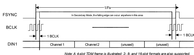
Figure 4-29. TDM Data Format—1 x DIN
