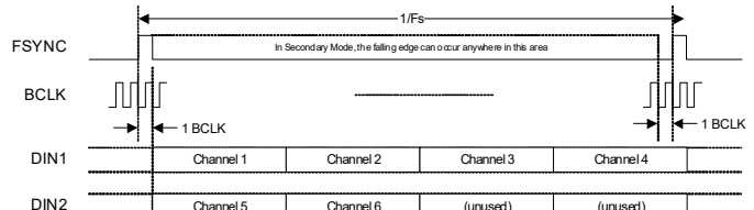
Figure 4-20. TDM Data Format—2 x DIN
