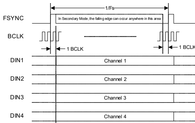
Figure 4-16. TDM Data Format—4 x DIN
