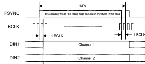
Figure 4-20. TDM Data Format—2 x DIN
