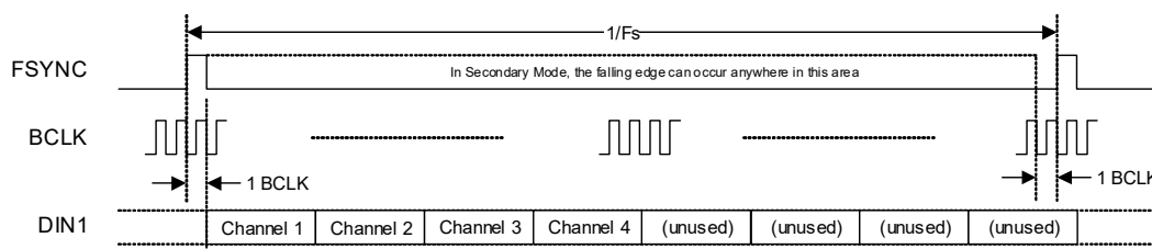
Figure 4-14. TDM Data Format—1 x DIN
