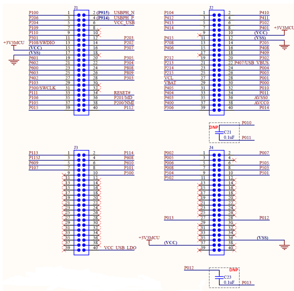
Figure 24. EK-RA4M1 Pin Headers Circuits
