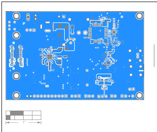
MAX96717/MAX96793 EV Kit—Bottom
