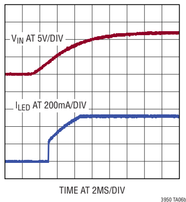
Startup Using Always-On Input
