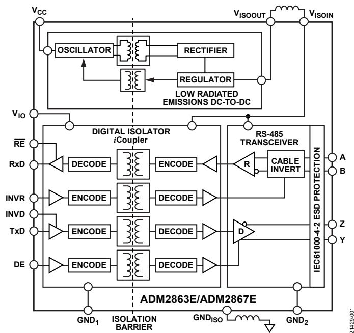
Figure 1. ADM2863E/ADM2867E
