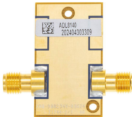
Figure 2. ADL8140-EVALZ Bottom
