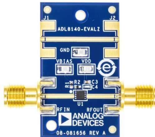
Figure 1. ADL8140-EVALZ Top
