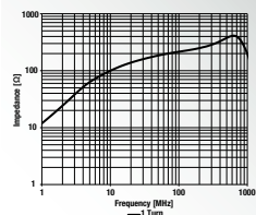
782 013 068 250 Ø Cable: 6.8 mm Material: 1E04_620
