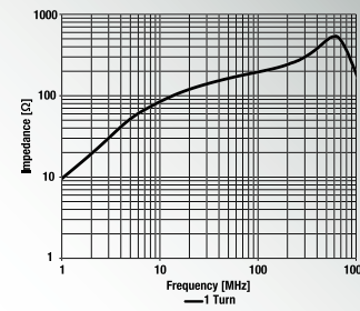
782 013 150 285 Ø Cable: 15.0 mm Material: 1E04_620
