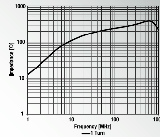
782 013 125 285 Ø Cable: 12.5 mm Material: 1E04_620
