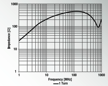
782 013 076 508 Ø Cable: 7.6 mm Material: 1E04_620
