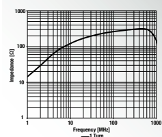
782 013 046 250 Ø Cable: 4.6 mm Material: 1E04_620
