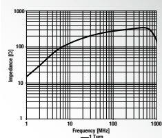
782 013 069 285 Ø Cable: 6.9 mm Material: 1E04_620
