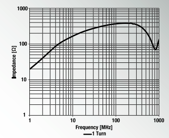
782 013 057 450 Ø Cable: 5.7 mm Material: 1E04_620
