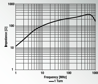
782 013 091 285 Ø Cable: 9.1 mm Material: 1E04_620
