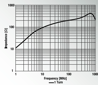
782 013 086 280 Ø Cable: 8.6 mm Material: 1E04_620
