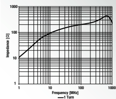
782 013 079 285 Ø Cable: 7.9 mm Material: 1E04_620
