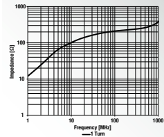
782 013 033 150 Ø Cable: 3.3 mm Material: 1E04_620
