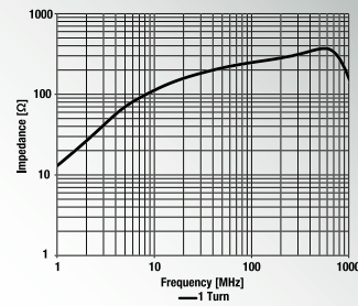
782 013 076 285 Ø Cable: 7.6 mm Material: 1E04_620
