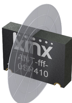
YZ-Plane Gain
