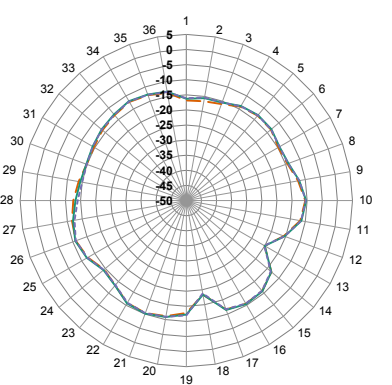
YZ-Plane Gain
