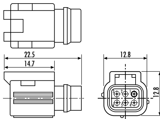
RECEPTACLE - TYPE 1
