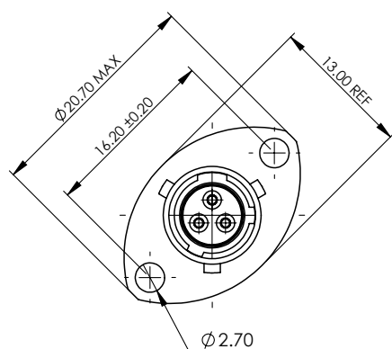
RECEPTACLE - TYPE 0
