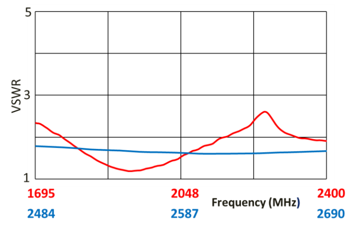
VSWR
