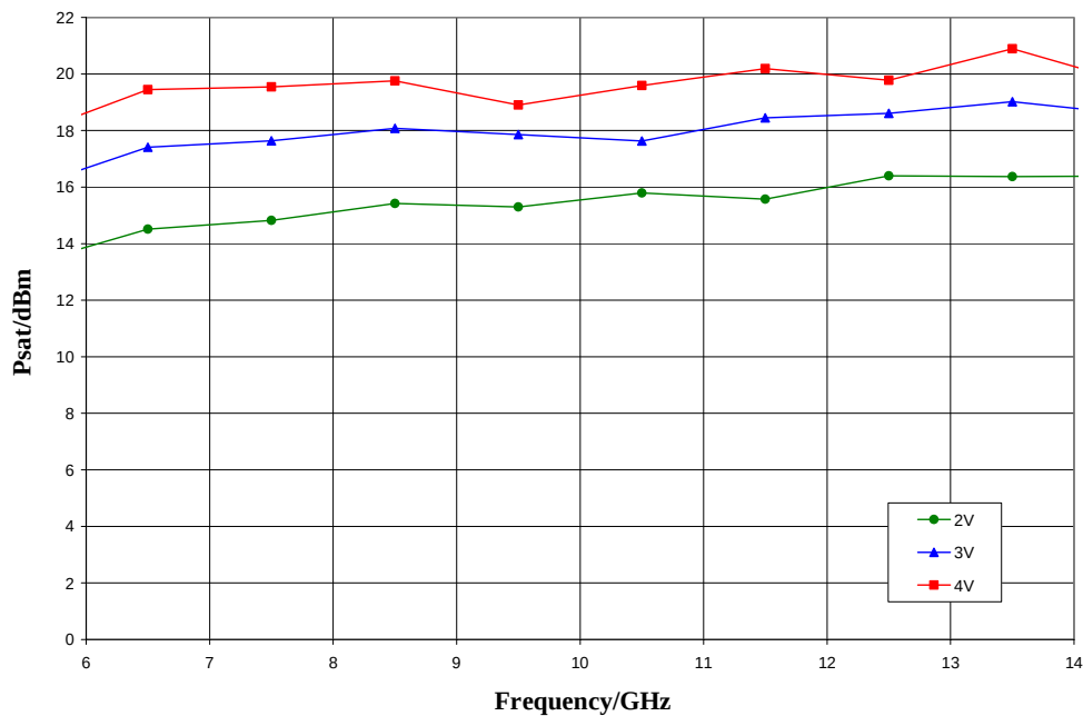
Psat vs. V_{dd} , V_{gg}=1.5\text{ V} , T_A=25\text{ °C}
