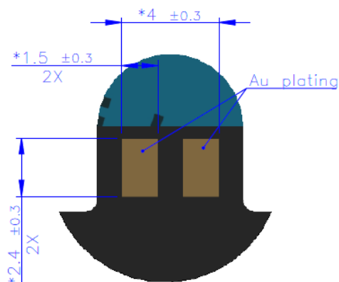
Detail A 5 : 1
