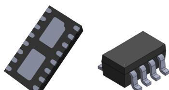
QFN-16L 4.0 x 2.0 x 0.9 mm SOT23-8L 2.9 x 2.8 mm
