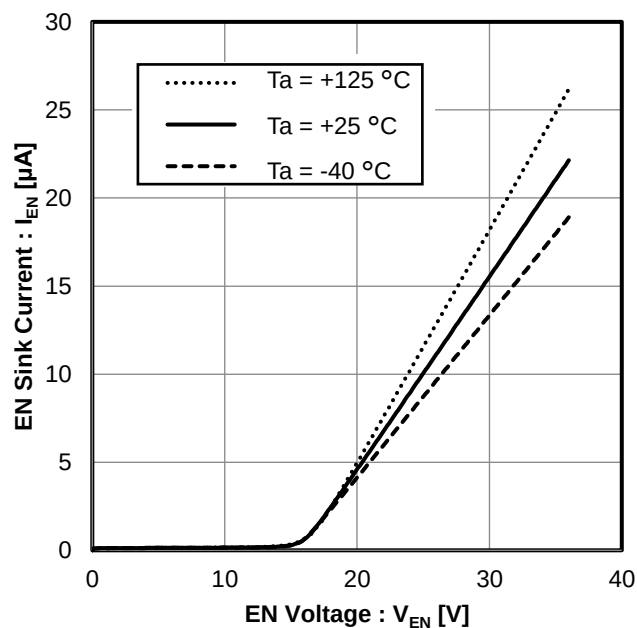
Figure 20. EN Sink Current vs EN Voltage
