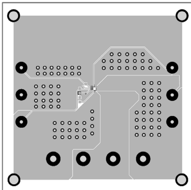
Figure2: Top Layer
