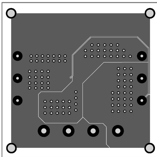
Figure3: Bottom Layer
