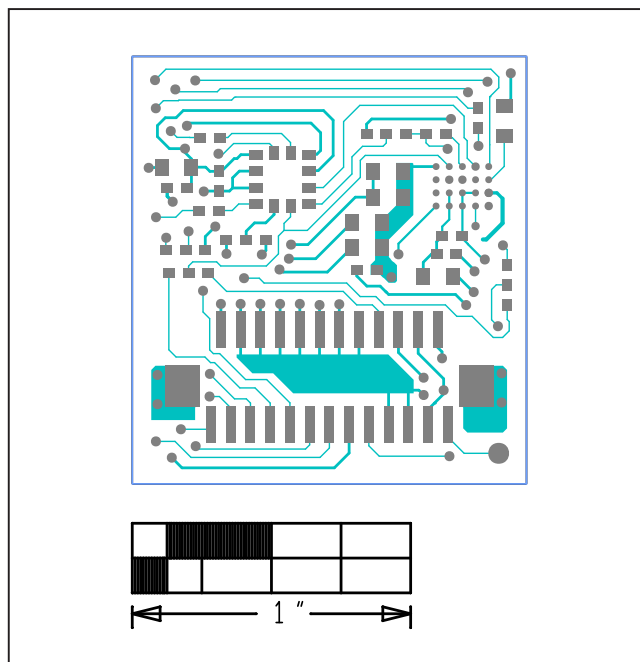
MAX86141OSBEK#—Top
