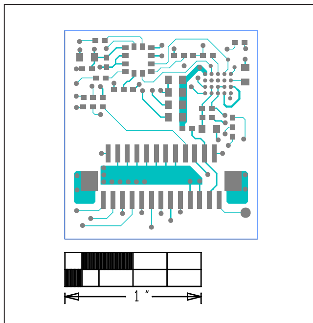
MAX86140OSBEK#—Top
