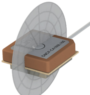
YZ-Plane Gain
