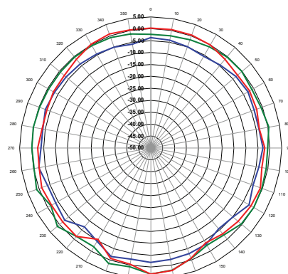
XZ-Plane Gain
