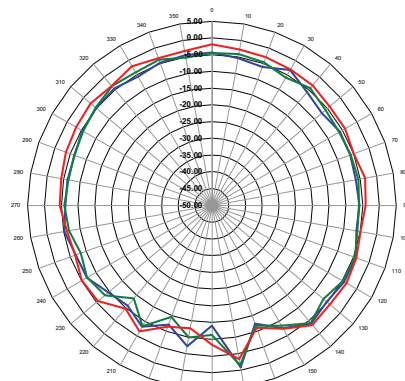
XZ-Plane Gain
