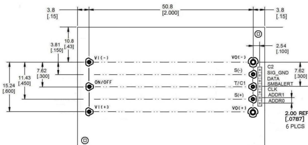
BOTTOM VIEW***
