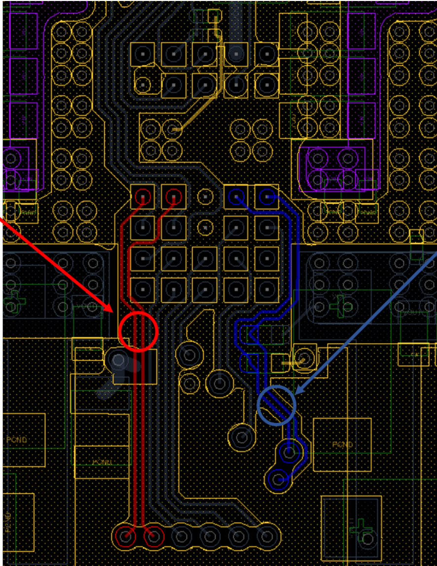
Figure 33 : VSense Traces
