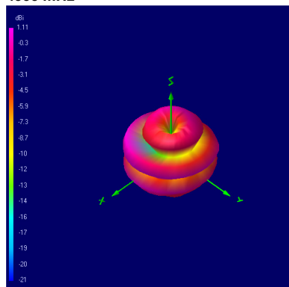
4900 MHz
