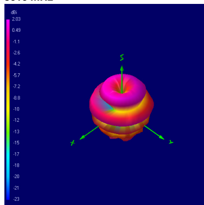
5016 MHz
