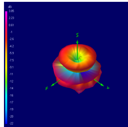
5512 MHz
