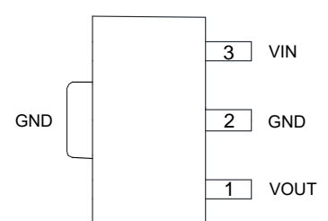
SOT89
