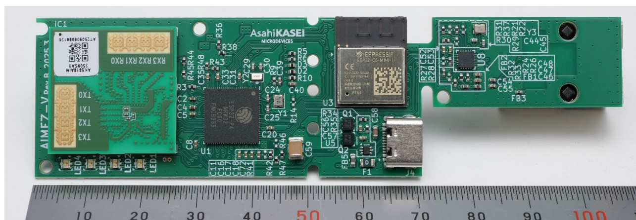
Fig.1.3.1.1. Top view
