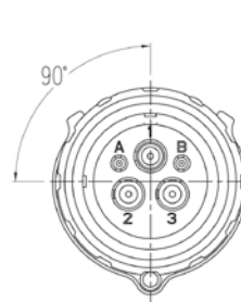
STRAIGHT PLUG STECKER, GERADE CONNECTEUR DROIT
